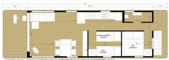
RALPHÖHE: 212,5cm HOHE DES HAUSBOOTS (VON DER UNTERSEITE DES FLOATS BIS ZUR DACHBEREITE): 340,5cm
